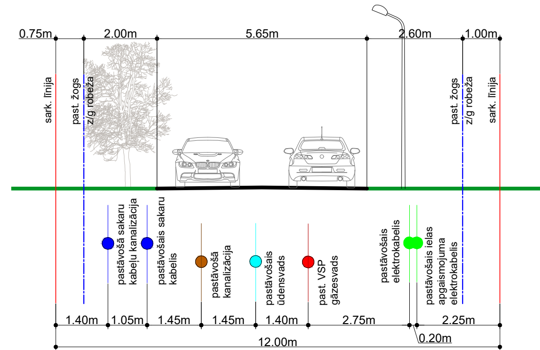
Braslas iela, sarkanās līnijas 12,0m, E kategorijas iela, griezumums B-B
